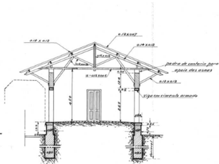
Corte por A.B.
